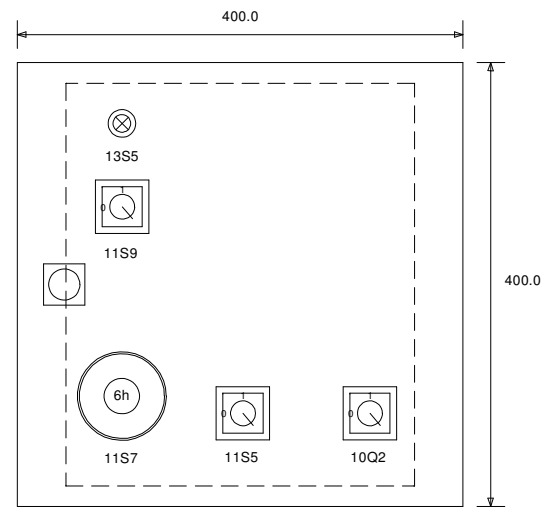
SCHAKELKAST VOOR-AANZICHT
